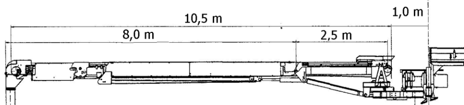
Vista de lado : PLEGADA SOBRE CAMIÓN-OLLA
