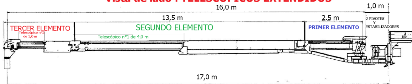
Vista de lado : TELESCÓPICOS EXTENDIDOS
