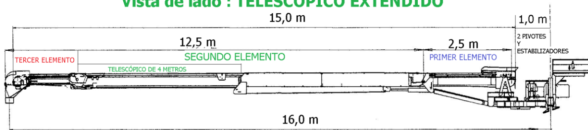
Vista de lado : TELESCÓPICO EXTENDIDO
