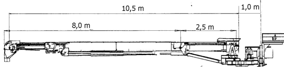
Vista de lado : PLEGADA SOBRE CAMIÓN-OLLA.
